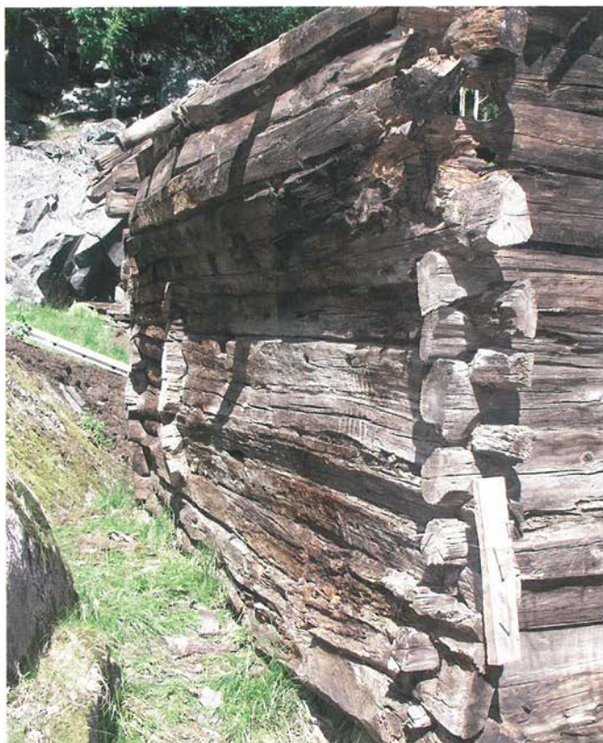
Stokkane har vridd seg kraftig i veggens mot vest. Dette skuldast delvis at novhovuda er skada.
