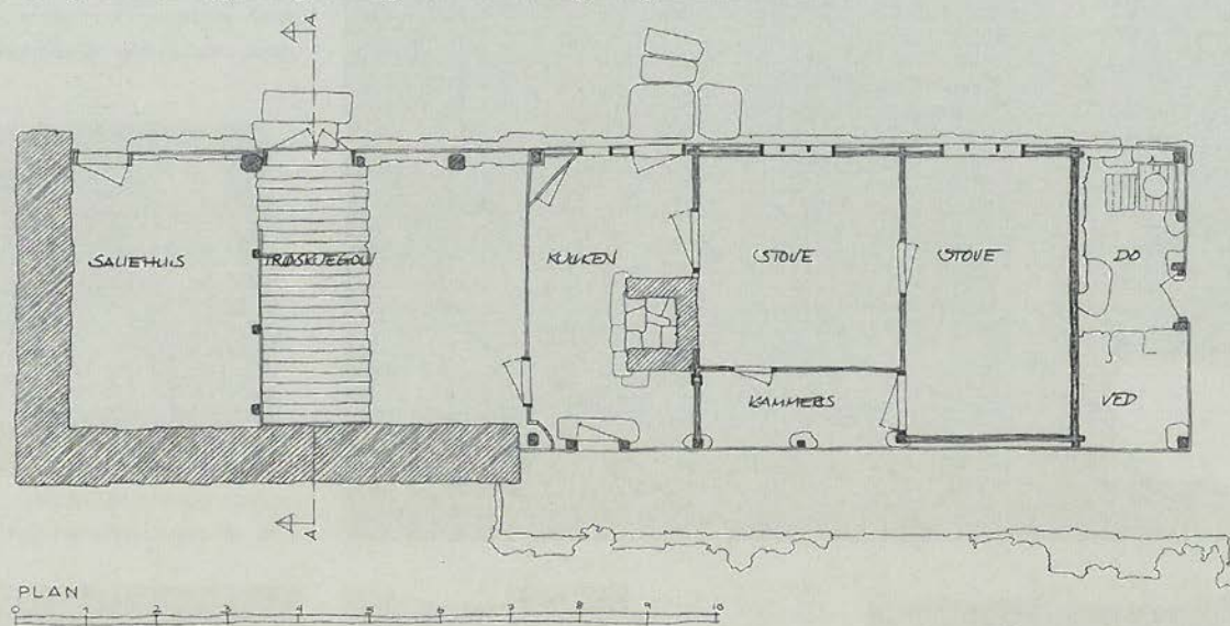
Planteikning av huset på Bakken. Oppmålingsteikning ved Helliesen og Waage arkitektkontor.
